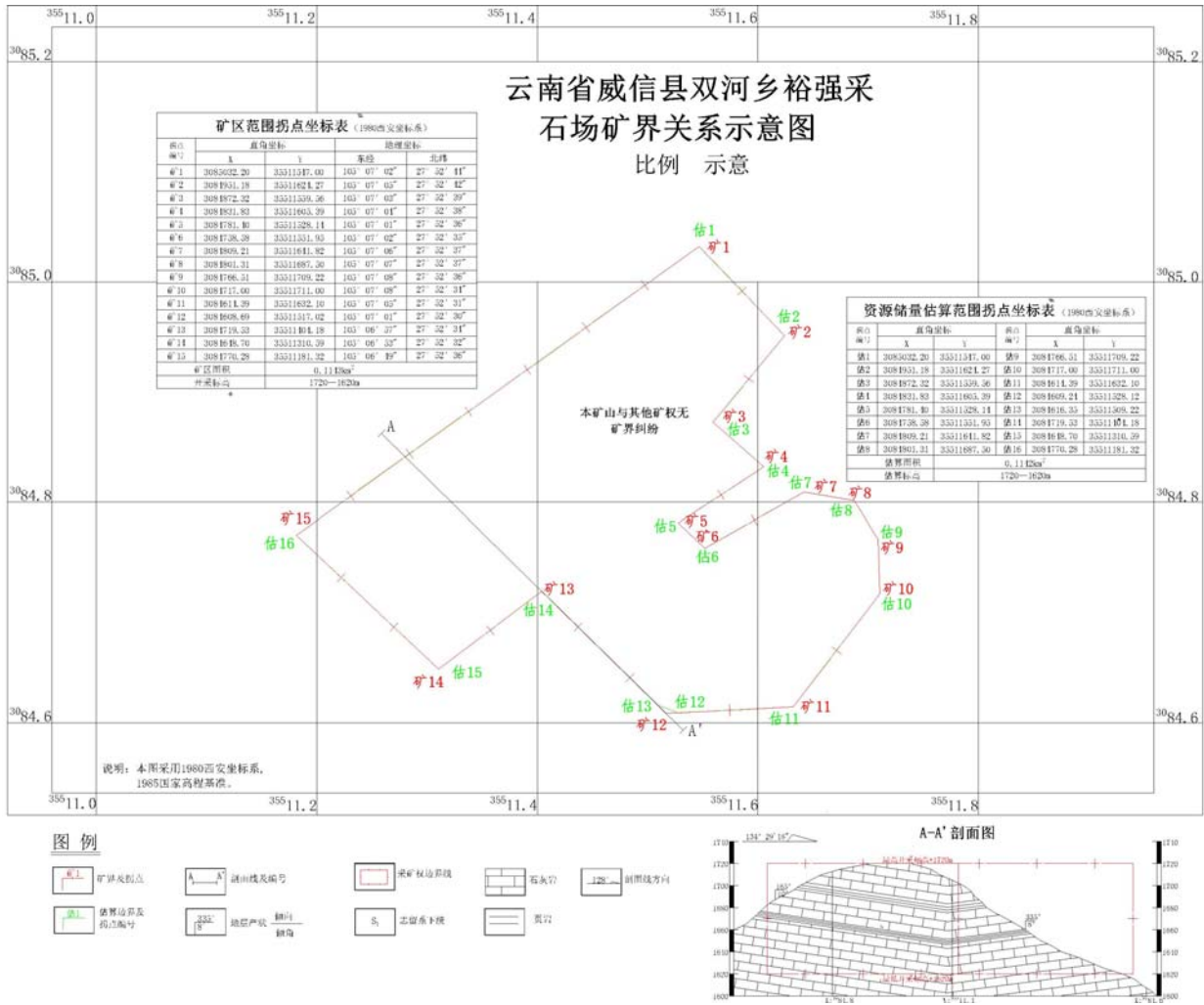
图1 矿产资源储量估算范围与划定矿区范围的位置关系图
